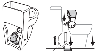
S-trap Connector ข้อต่อทางน้ำเสียแบบลงพื้น
