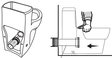
P-trap Connector ข้อต่อทางน้ำเสียแบบออกผนัง
