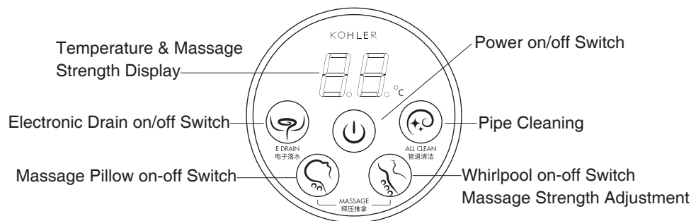
Keypad Type 2
