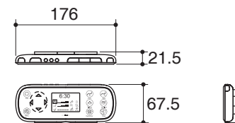
รีโมทคอนโทรล
