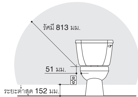
ระยะการติดตั้งอุปกรณ์ไฟฟ้า
