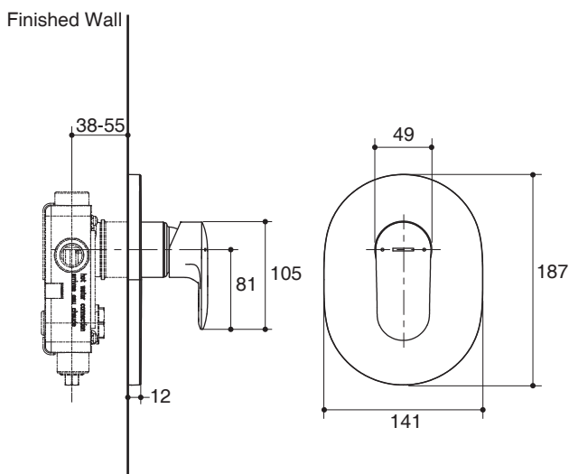
K-99471T-4
