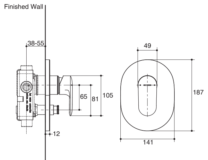
K-99472T-4
