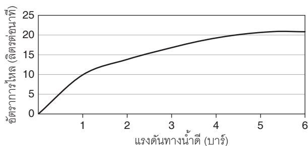
กราฟแสดงอัตราการไหล ก๊อกกลางแจ้ง
